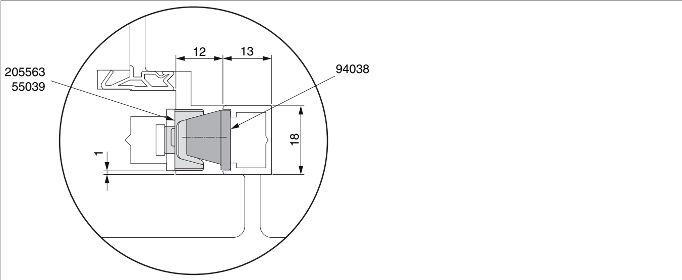
Detailansicht mit Schließzapfen für gegenüberliegende Beschlagsnut
