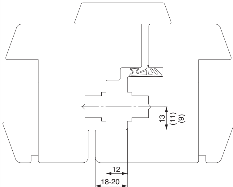
Gegenüberliegende Beschlagsnut mit Alukanal
