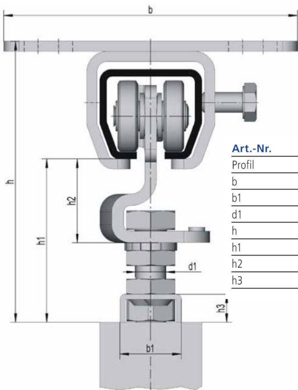
Abbildung 2. Einbauschnitt mit den Rollapparaten
