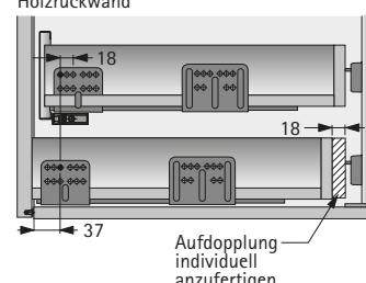
Holzurückwand
