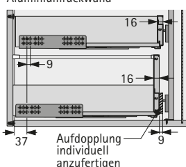
Aluminiumrückwand
