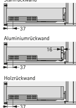
Schubkasten / Frontauszug mit Stahlrückwand
