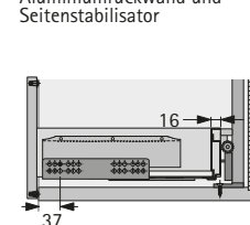
Schubkasten / Frontauszug mit Stahl- oder Aluminiumrückwand und Seitenstabilisator
