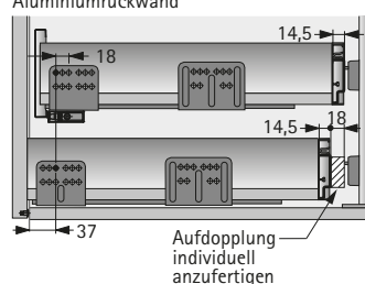
Aluminiumrückwand
