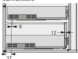
Innenschubkasten / -auszug mit Stahlrückwand
