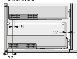
Holzurückwand
