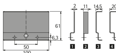
Aluminiumrückwand
