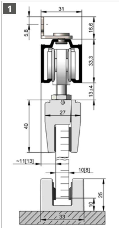
HELM 73 – Wandmontage, mit Wandwinkel 61/01 Beschlagzusammenstellung siehe Seite 26
