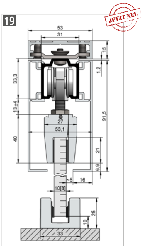
HELM 73 WT – Wandtaschenmontage mit Befestigungsschiene Beslagzusammenstellung siehe Seite 30
