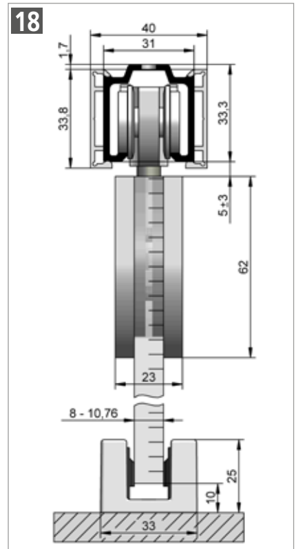
HELM 73 – Deckenmontage, mit beidseitiger ME Verblendung der Laufschiene und Flansch mit Verblendung für ESG/VSG Glas Beschlagzusammenstellung siehe Seite 30
