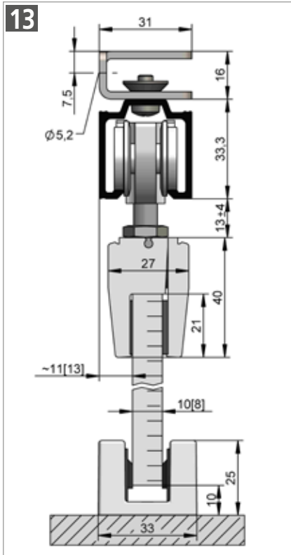
HELM 73 WT – Wandtaschenmontage mit Wandbügel bzw. Deckenbügel Beschlagzusammenstellung siehe Seite 29
