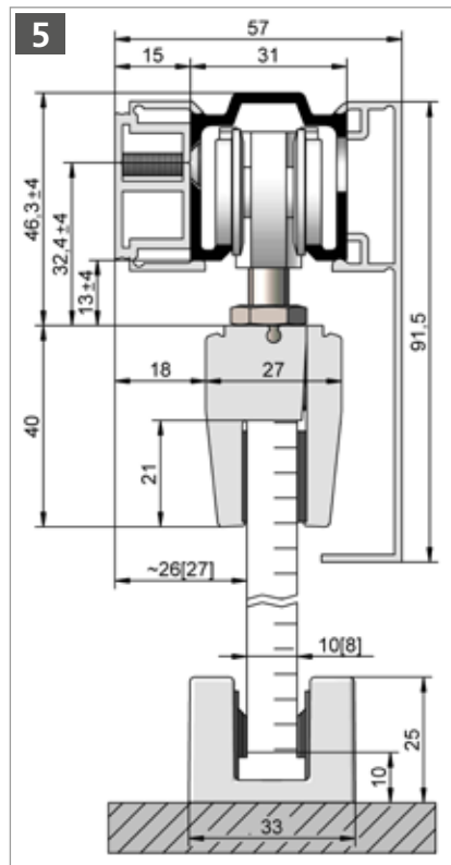
HELM 73 – Wandmontage, mit seitlich gebohrter Laufschiene, Abstandsprofil einseitig und einseitiger Verblendung Beschlagzusammenstellung siehe Seite 27
