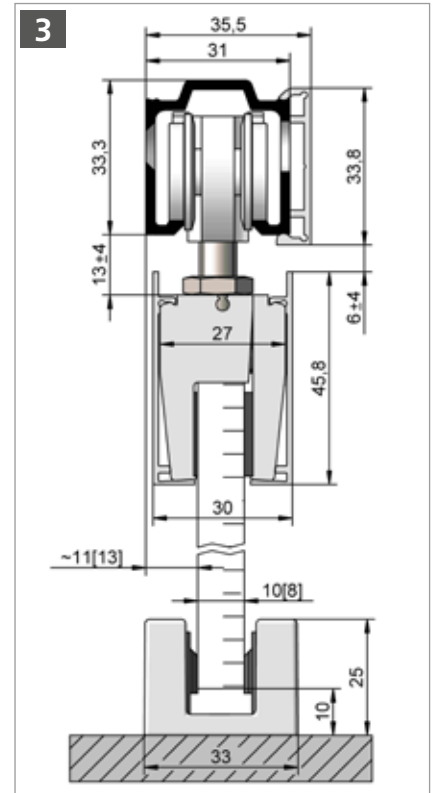
HELM 73 – Wandmontage, mit seitlich gebohrter Laufschiene, einseitige ME Verblendung der Lauf- schiene und Verblendung der Glasklemmstücke Beschlagzusammenstellung siehe Seite 26
