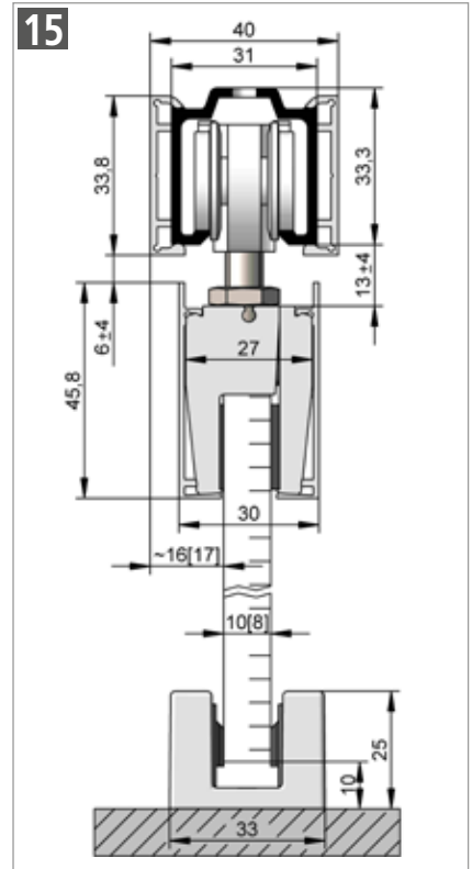
HELM 73 – Deckenmontage, mit beidseitiger ME Verblendung der Laufschiene und Verblendung der Glasklemmstücke Beschlagzusammenstellung siehe Seite 30
