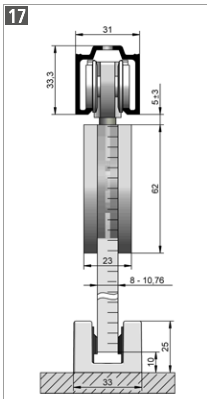
HELM 73 – Deckenmontage, Flansch mit Verblendung für ESG/VSG Glas Beschlagzusammenstellung siehe Seite 30
