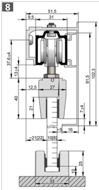
HELM 73 – Wandmontage , mit Montageschiene und einseitiger Verblendung Beschlagzusammenstellung siehe Seite 27
