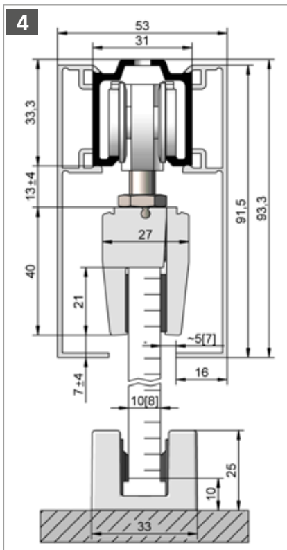
HELM 73 – Deckenmontage, mit beidseitiger Verblendung Beschlagzusammenstellung siehe Seite 26
