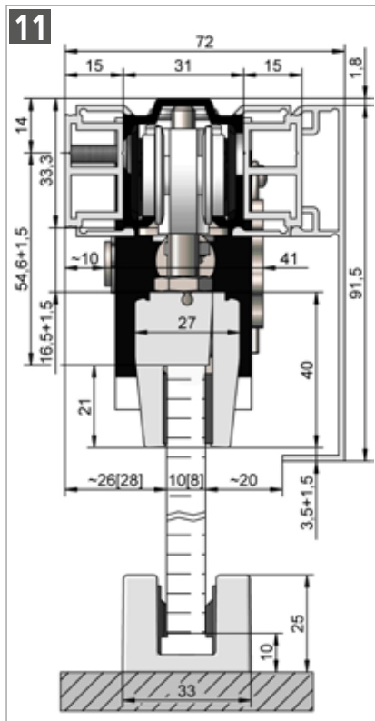
HELM 73 – Wandmontage , SmartStop/SmartClose mit seitlich gebohrter Laufschiene, Abstandsprofil beidseitig und einseitiger Verblendung Beschlagzusammenstellung siehe Seite 28
