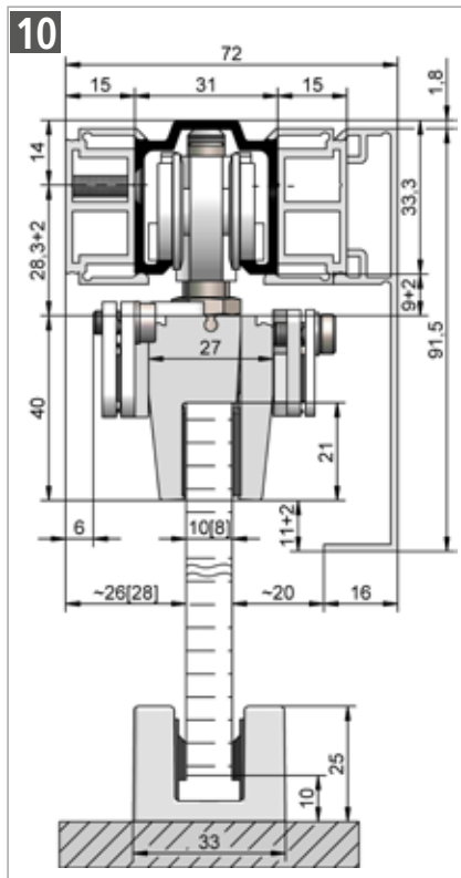
HELM 73 – Wandmontage , synchron mit seitlich gebohrter Laufschiene, Abstandsprofil beidseitig und einseitiger Verblendung Beschlagzusammenstellung siehe Seite 28
