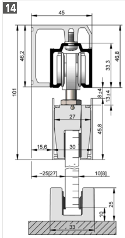
HELM 73 – Wandmontage, mit Montage-schiene und Verblendung der Glasklemmstücke Beschlagzusammenstellung siehe Seite 30
