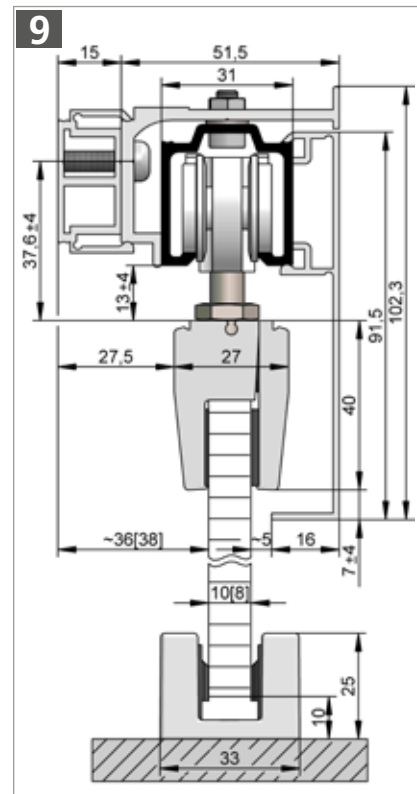
HELM 73 – Wandmontage , mit Abstandsprofil, Montageschiene und einseitiger Verblendung Beschlagzusammenstellung siehe Seite 28
