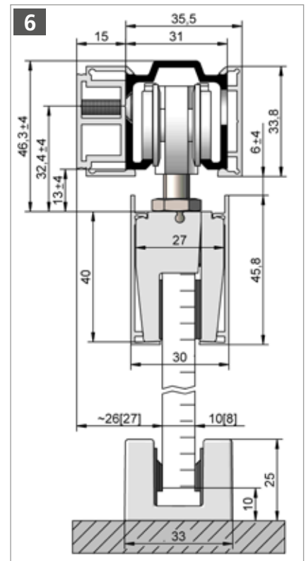
HELM 73 – Wandmontage, mit seitlich gebohrter Laufschiene, Abstandsprofil, einseitiger ME Verblendung und Verblendung der Glasklemmstücke Beschlagzusammenstellung siehe Seite 27
