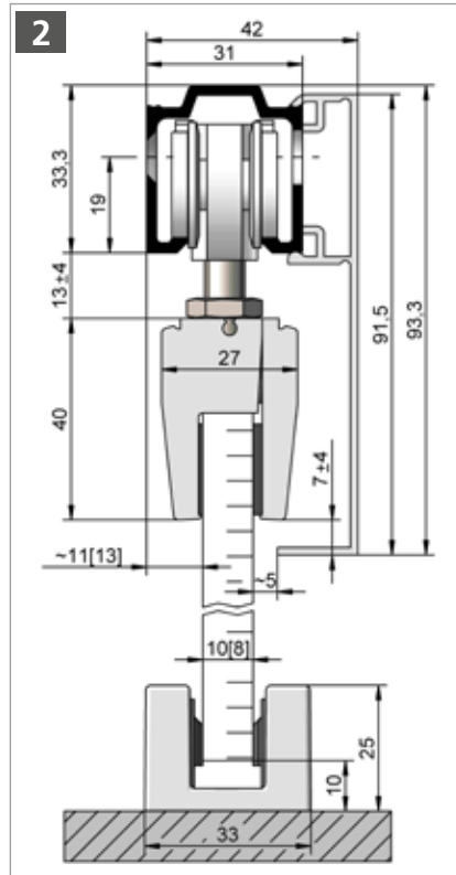
HELM 73 – Wandmontage, mit seitlich gebohrter Laufschiene und einseitiger Verblendung Beschlagzusammenstellung siehe Seite 26
