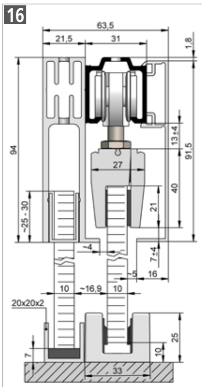
HELM 73 – Deckenmontage, mit Aufnahmeprofil für Festteil und einseitiger Verblendung Beschlagzusammenstellung siehe Seite 30
