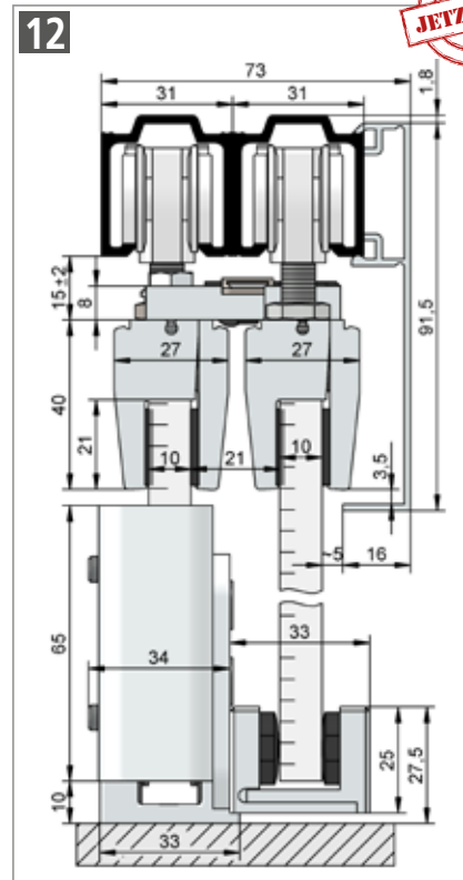
HELM 73 – Deckenmontage , Teleskopbeschlag mit HELM SmartGuide G und untere Führung zweigeteilt Beschlagzusammenstellung siehe Seite 29
