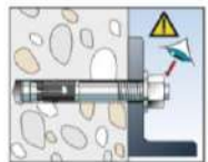
4: Position prüfen: Ein Gewindegang Überstand über die Mutter
