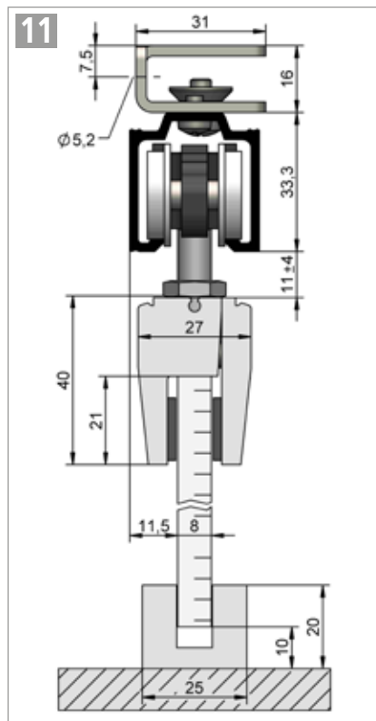
HELM 53 WT – Wandtaschenmontage , mit Wandbügel bzw. Deckenbügel Beschlagzusammenstellung siehe Seite 29
