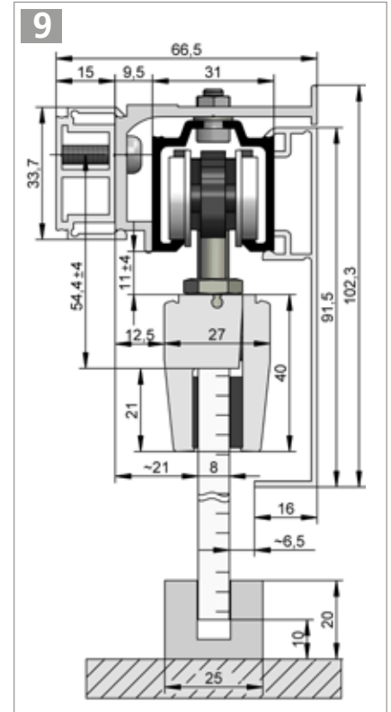
HELM 53 – Wandmontage , mit Abstandsprofil, Montageschiene und einseitiger Verblendung Beschlagzusammenstellung siehe Seite 28
