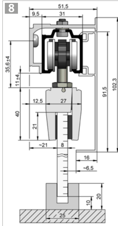
HELM 53 – Wandmontage , mit Montageschiene und einseitiger Verblendung Beschlagzusammenstellung siehe Seite 27
