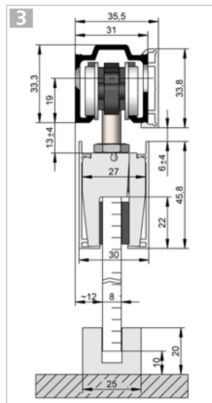
HELM 53 – Wandmontage, mit seitlich gebohrter Laufschiene und einseitiger ME Verblendung und Verblendung der Glasklemmstücke Beschlagzusammenstellung siehe Seite 26
