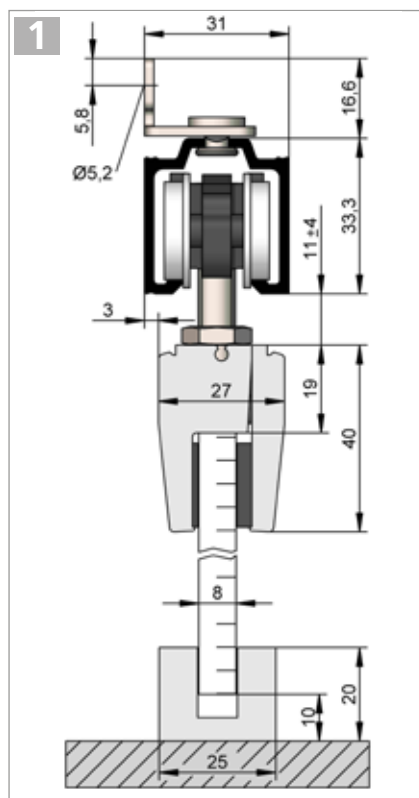
HELM 53 – Wandmontage, mit Wandwinkel 61/01 Beschlagzusammenstellung siehe Seite 26
