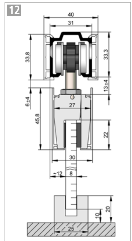
HELM 53 – Deckenmontage , mit beidseitiger ME Verblendung der Laufschiene und Verblendung der Glasklemmstücke Beschlagzusammenstellung siehe Seite 30
