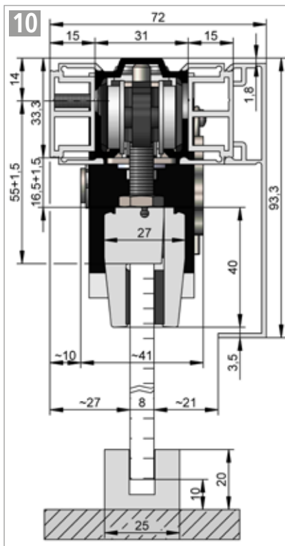
HELM 53 – Wandmontage , SmartStop/SmartClose mit seitlich gebohrter Laufschiene, Abstandsprofil beidseitig und einseitiger Verblendung Beschlagzusammenstellung siehe Seite 28
