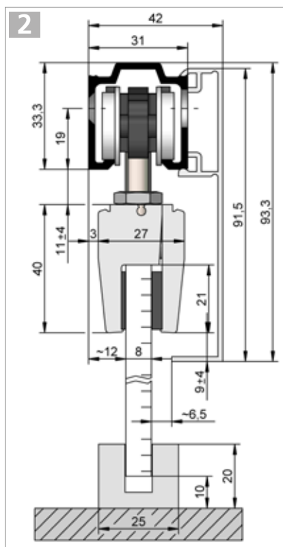
HELM 53 – Wandmontage, mit seitlich gebohrter Laufschiene und einseitiger Verblendung Beschlagzusammenstellung siehe Seite 26
