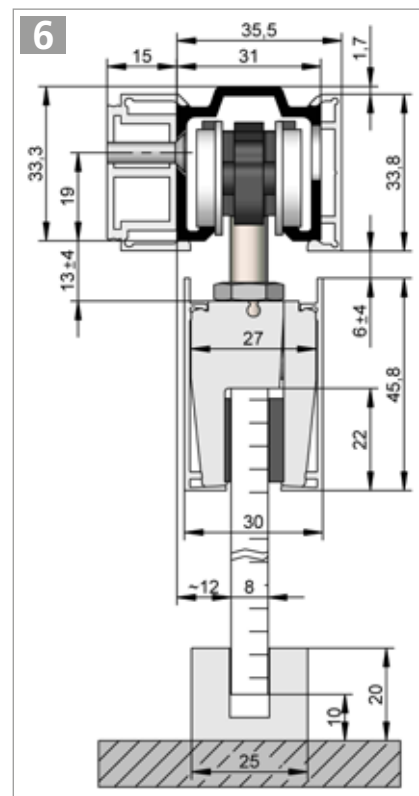
HELM 53 – Wandmontage, mit seitlich gebohrter Laufschiene, Abstandsprofil, einseitiger ME Verblendung und Verblendung der Glasklemmstücke Beschlagzusammenstellung siehe Seite 27
