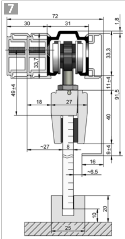
HELM 73 – Wandmontage , mit seitlich gebohrter Laufschiene, doppeltem Abstandsprofil und einseitiger Verblendung Beschlagzusammenstellung siehe Seite 27
