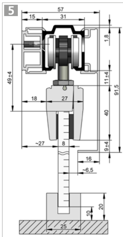
HELM 53 – Wandmontage, mit seitlich gebohrter Laufschiene, Abstandsprofil einseitig und einseitiger Verblendung Beschlagzusammenstellung siehe Seite 27
