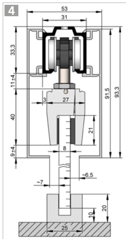
HELM 53 – Deckenmontage, mit beidseitiger Verblendung Beschlagzusammenstellung siehe Seite 26
