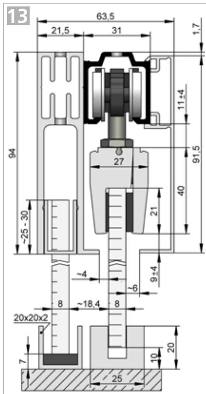
HELM 53 – Deckenmontage , mit Aufnahmeprofil für Festteil und einseitiger Verblendung Beschlagzusammenstellung siehe Seite 30
