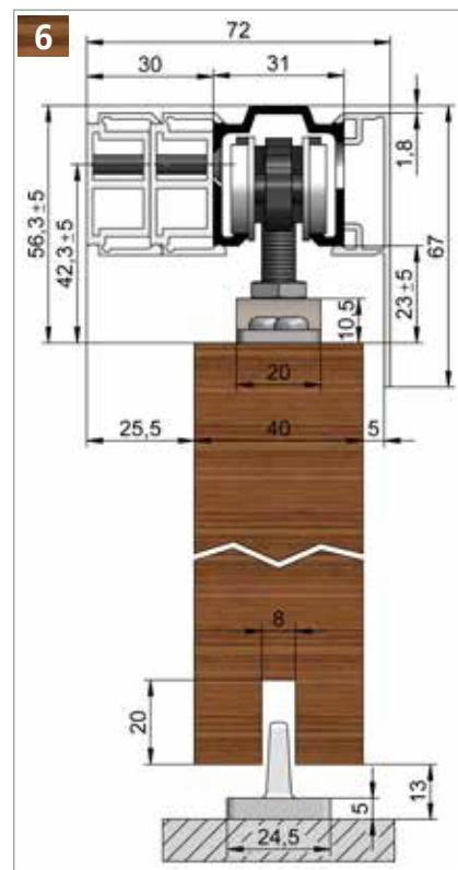
HELM 53 – Wandmontage, mit seitlich gebohrter Laufschiene, doppeltem Abstandsprofil und einseitiger Verblendung Beschlagzusammenstellung siehe Seite 27
