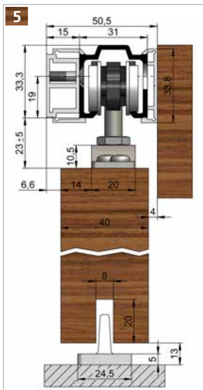
HELM 53 – Wandmontage, mit seitlich gebohrter Laufschiene, Abstandsprofil und einseitiger ME Verblendung (Holzverblendung bauseits) Beschlagzusammenstellung siehe Seite 27
