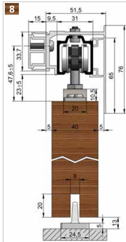
HELM 53 – Wandmontage , mit Montageschiene, Abstandsprofil und einseitiger Verblendung Beschlagzusammenstellung siehe Seite 28
