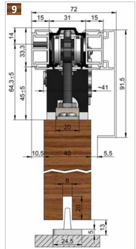
HELM 53 – Wandmontage , SmartStop/SmartClose mit seitlich gebohrter Laufschiene, Abstandsprofil beidseitig und einseitiger Verblendung Beschlagzusammenstellung siehe Seite 28
